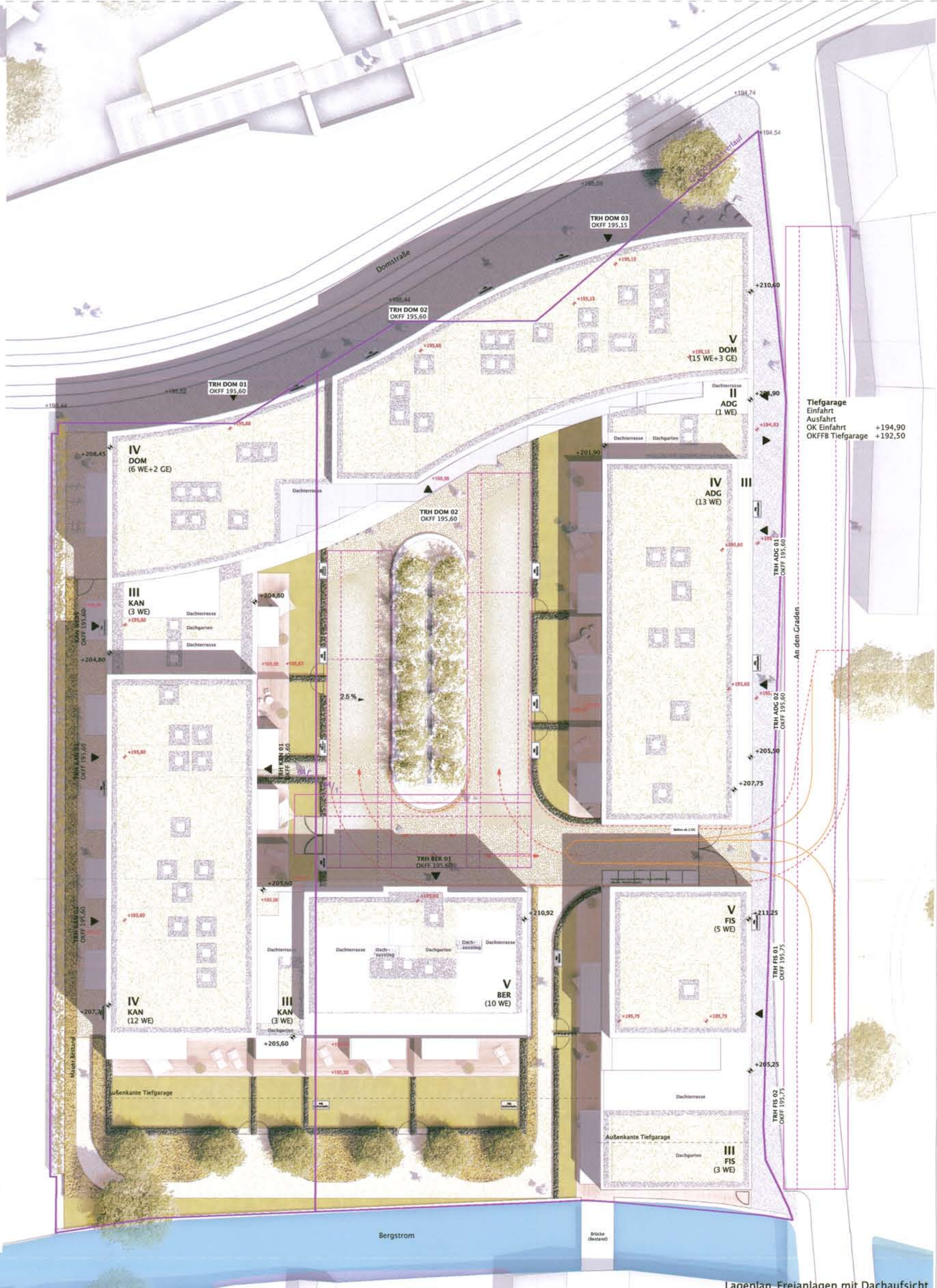
Lageplan-Freianlagen mit Dachaufsicht
