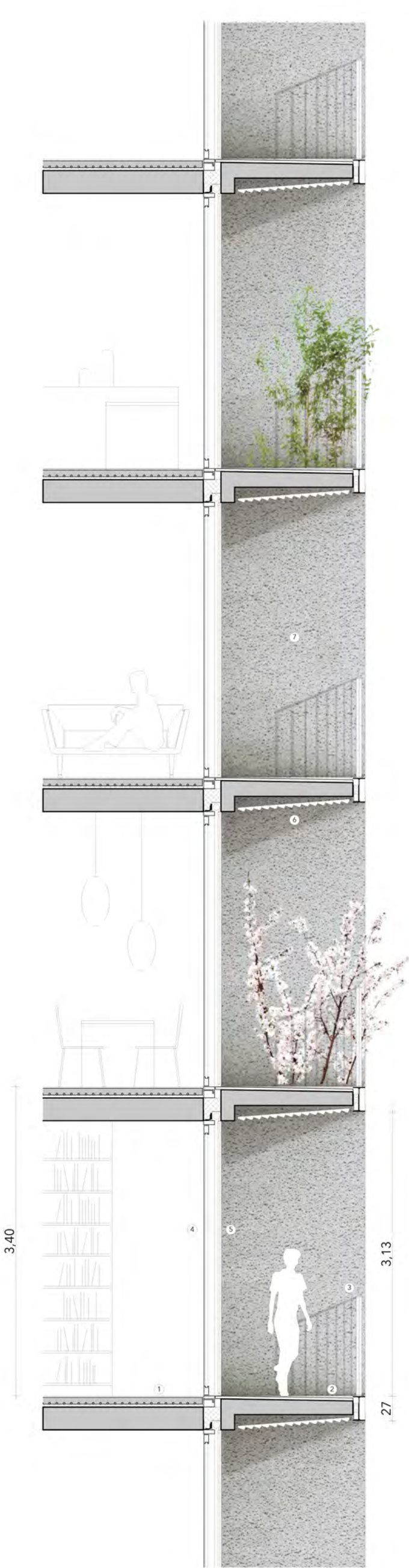
FASSADENSCHNITT M 1:50
