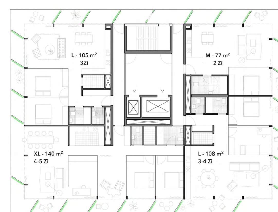
REGELGESCHOSS II 1:200 Familien, Gehoben und Senioren (unbetreut) 6.-9. OG im Wohnturm Norden 8.-9. OG im Wohnturm Süden
