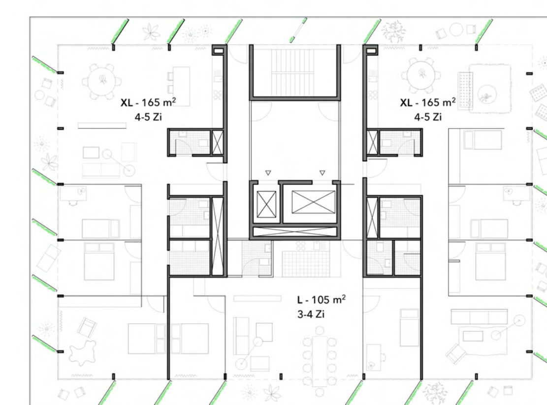
REGELGESCHOSS III 1:200 Gehoben und Familien 10.-15. OG im Wohnturm Norden
