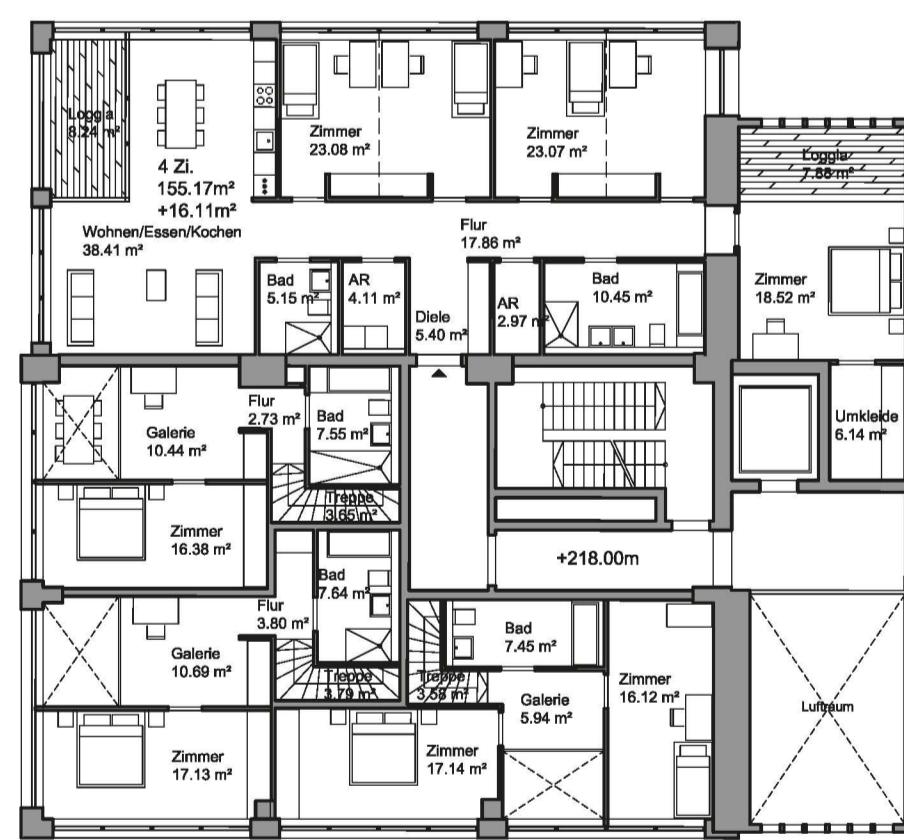
Grundriss 1.Obergeschoss Sudhaus_M 1:200
