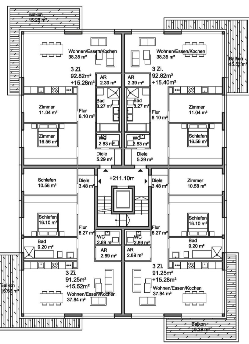
Grundriss RG1 Neubau_M 1:200
