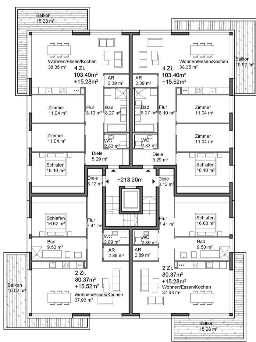
Grundriss RG2 Neubau_M 1:200
