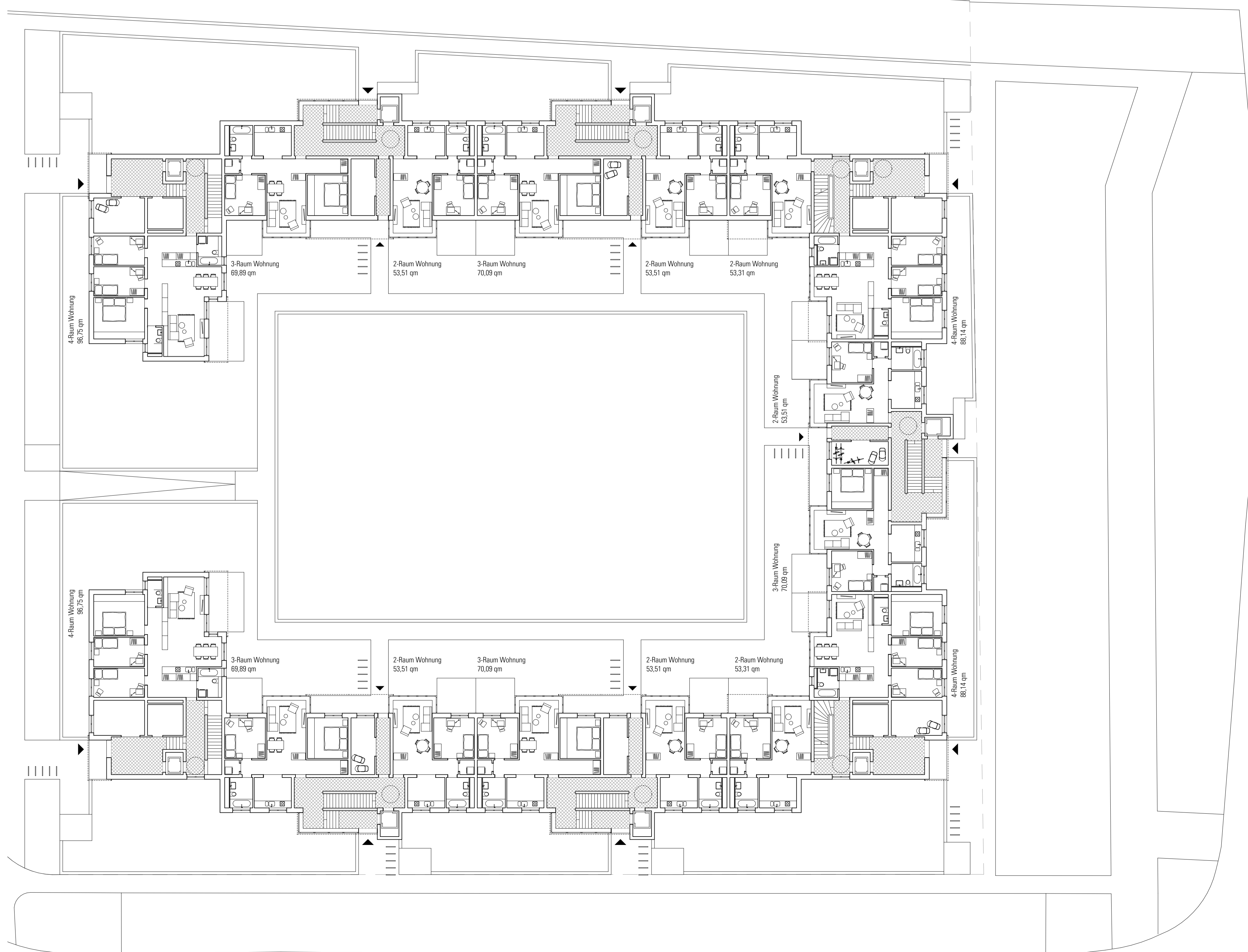
Erdgeschoss M 1:200
