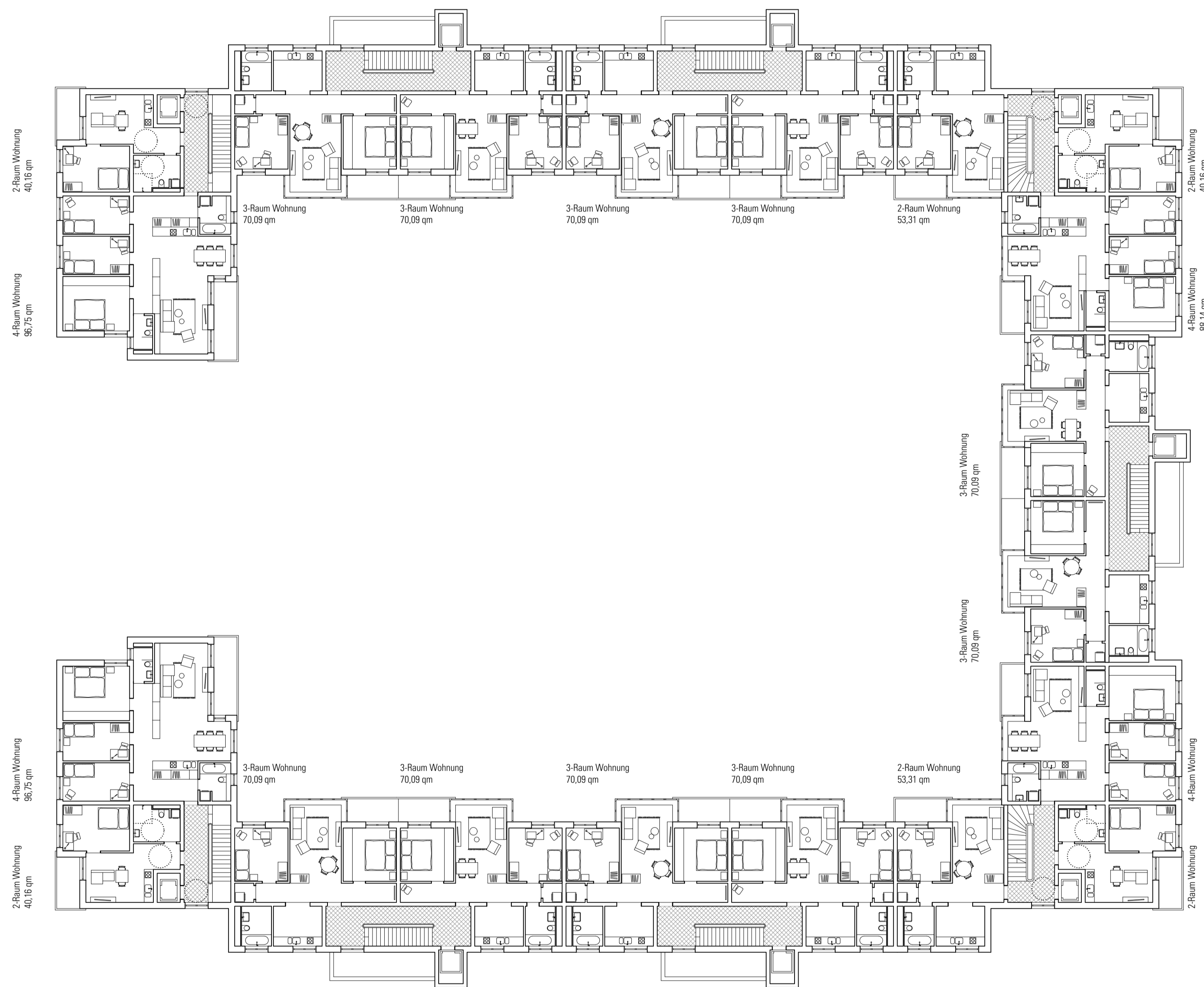
Regelgeschoss M 1:200
