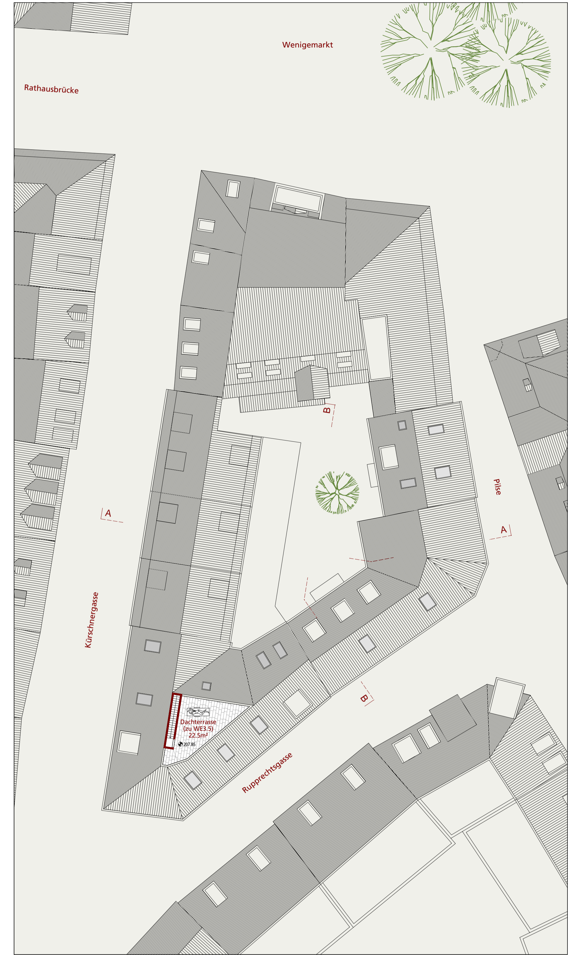
Grundriss Dachterrasse 1:200
