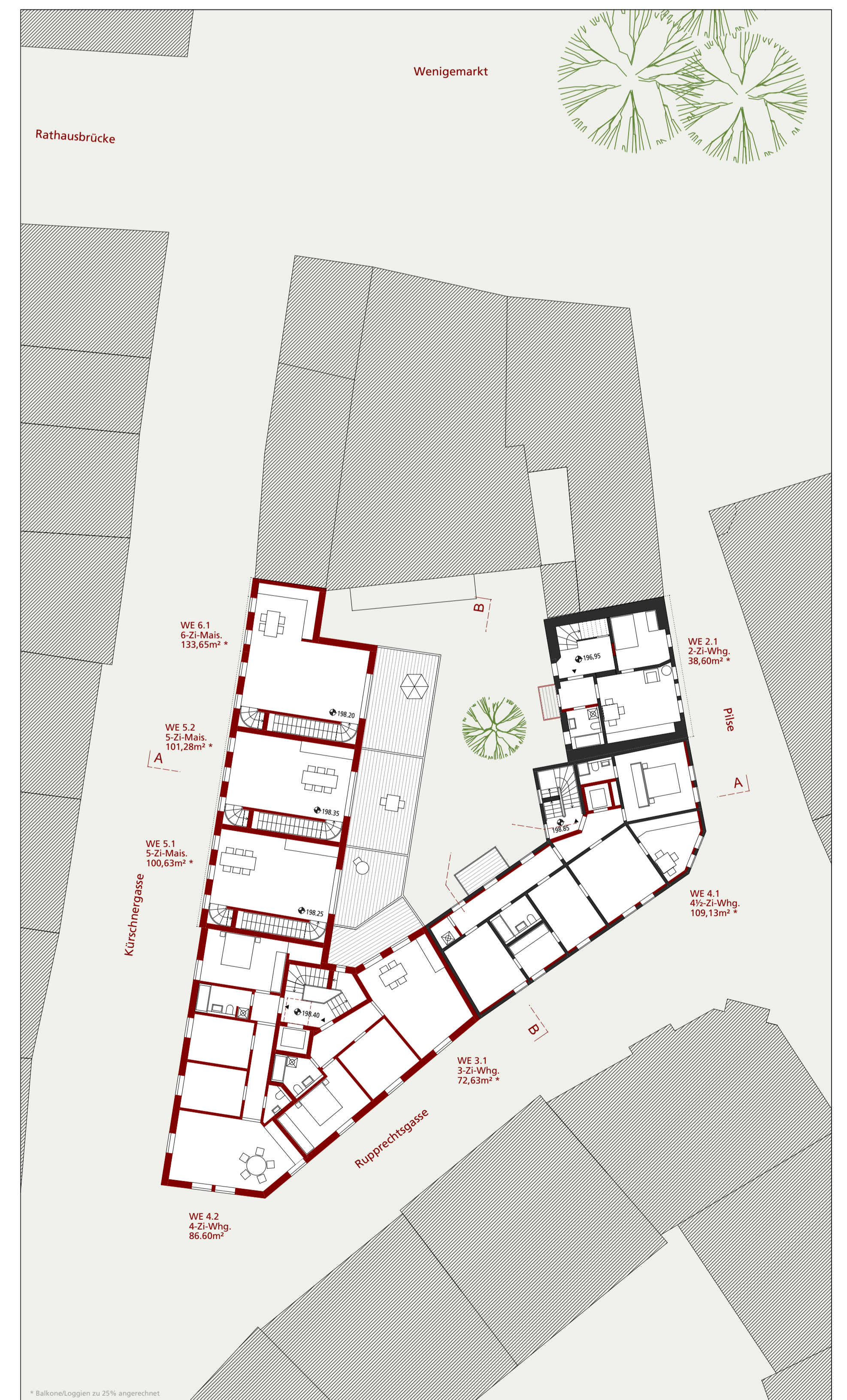
Grundriss 1.OG 1:200
