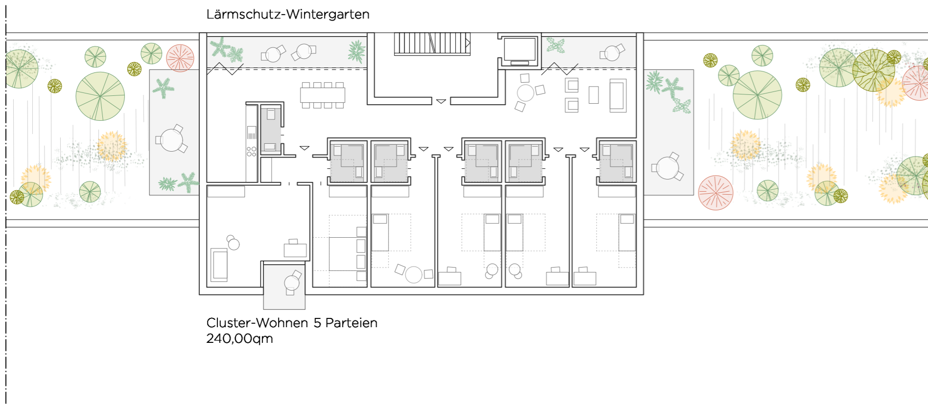
RG TEILBEREICH B GRUNDRISS LÄRMSCHUTZBEBAUUNG
