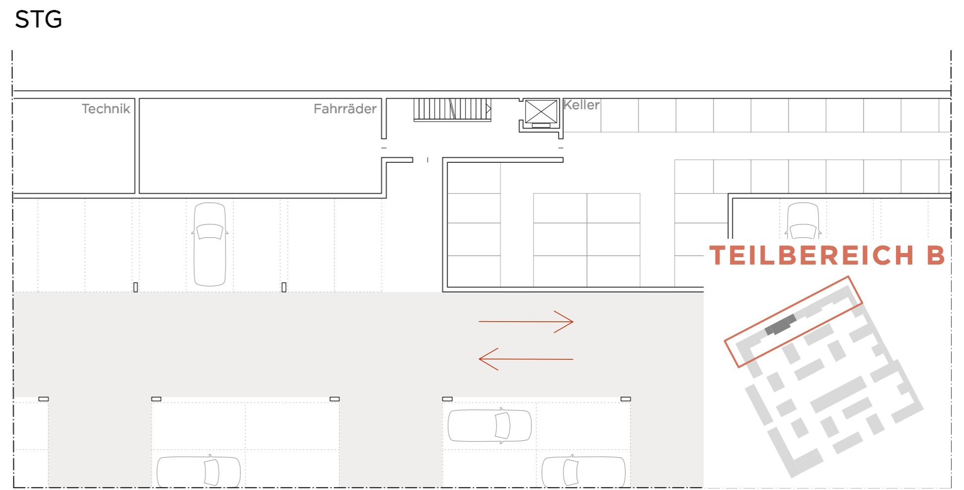
UG M 1:200
