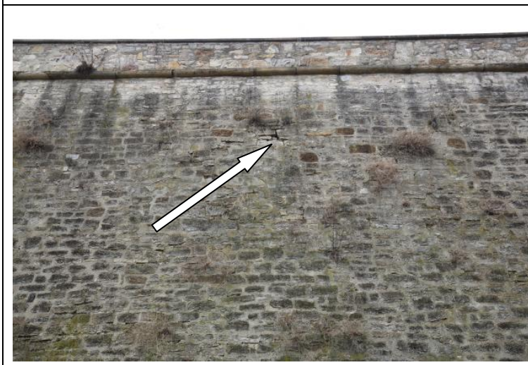
Abb. 17: Kleine Mauerwerksschäden
