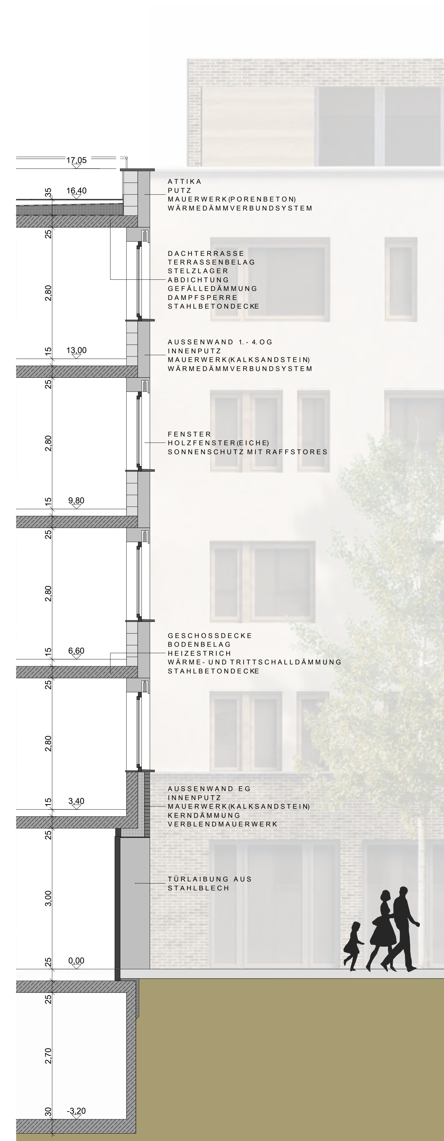
FASSADENSCHNITT M 1.50
