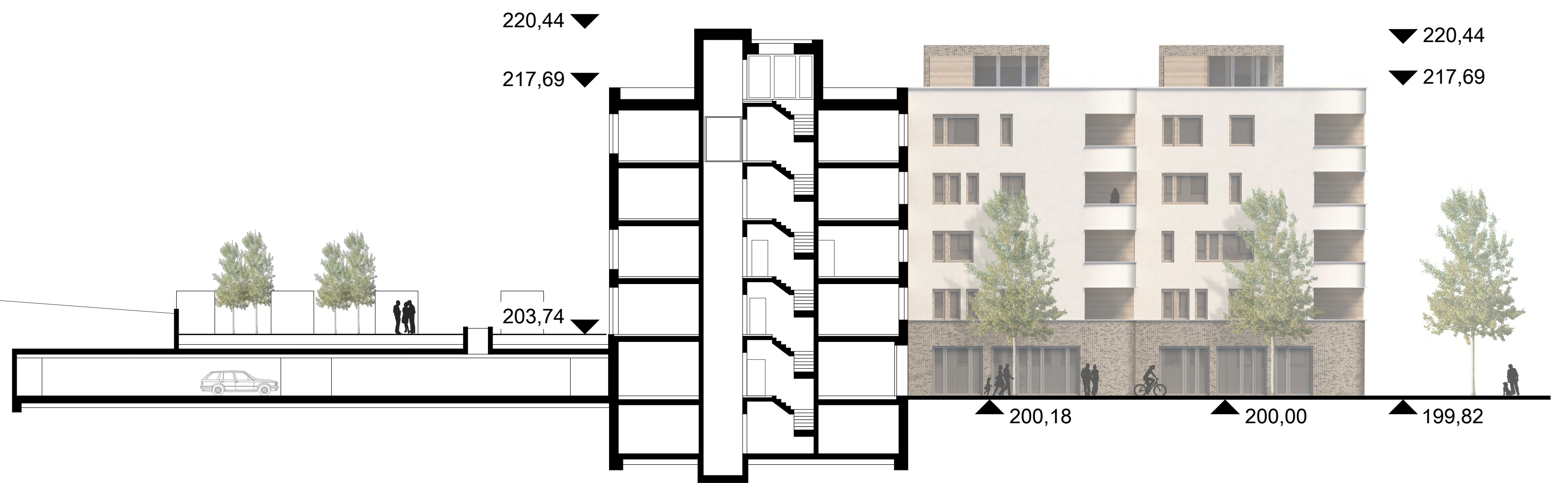
SCHNITT CC M 1.200
