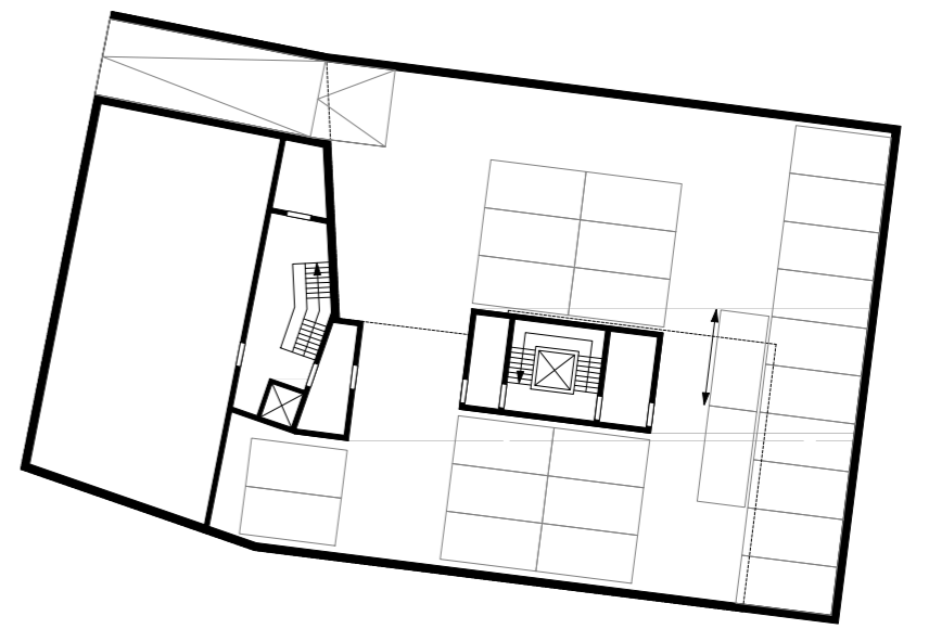
Grundriss Untergeschossebenen M 1:200
