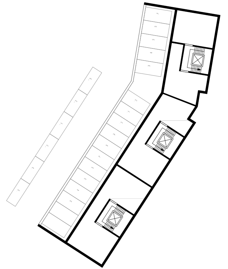
Grundriss Untergeschosse M 1:200
