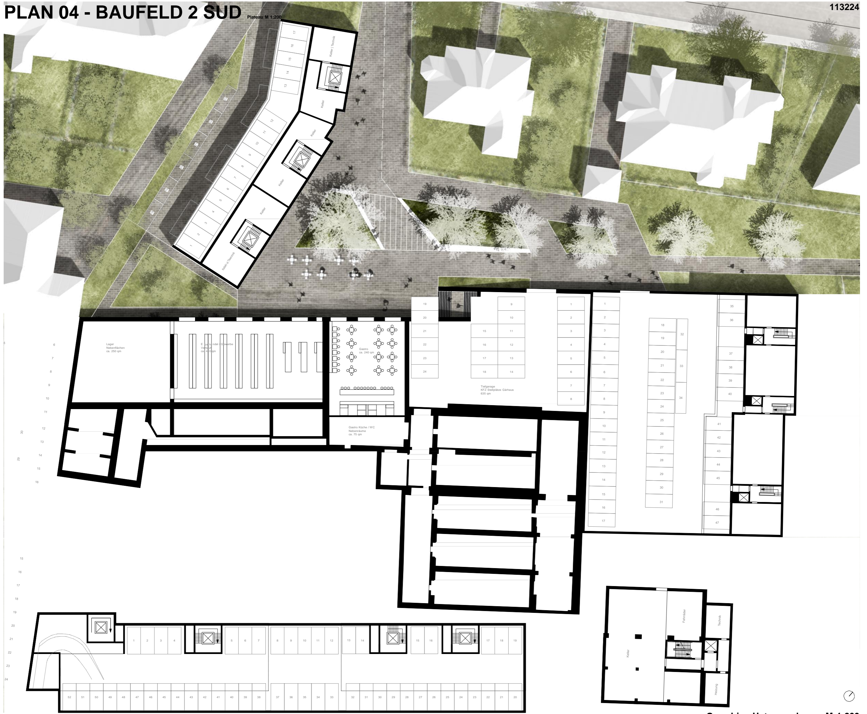
Grundriss Untergeschosse M 1:200
