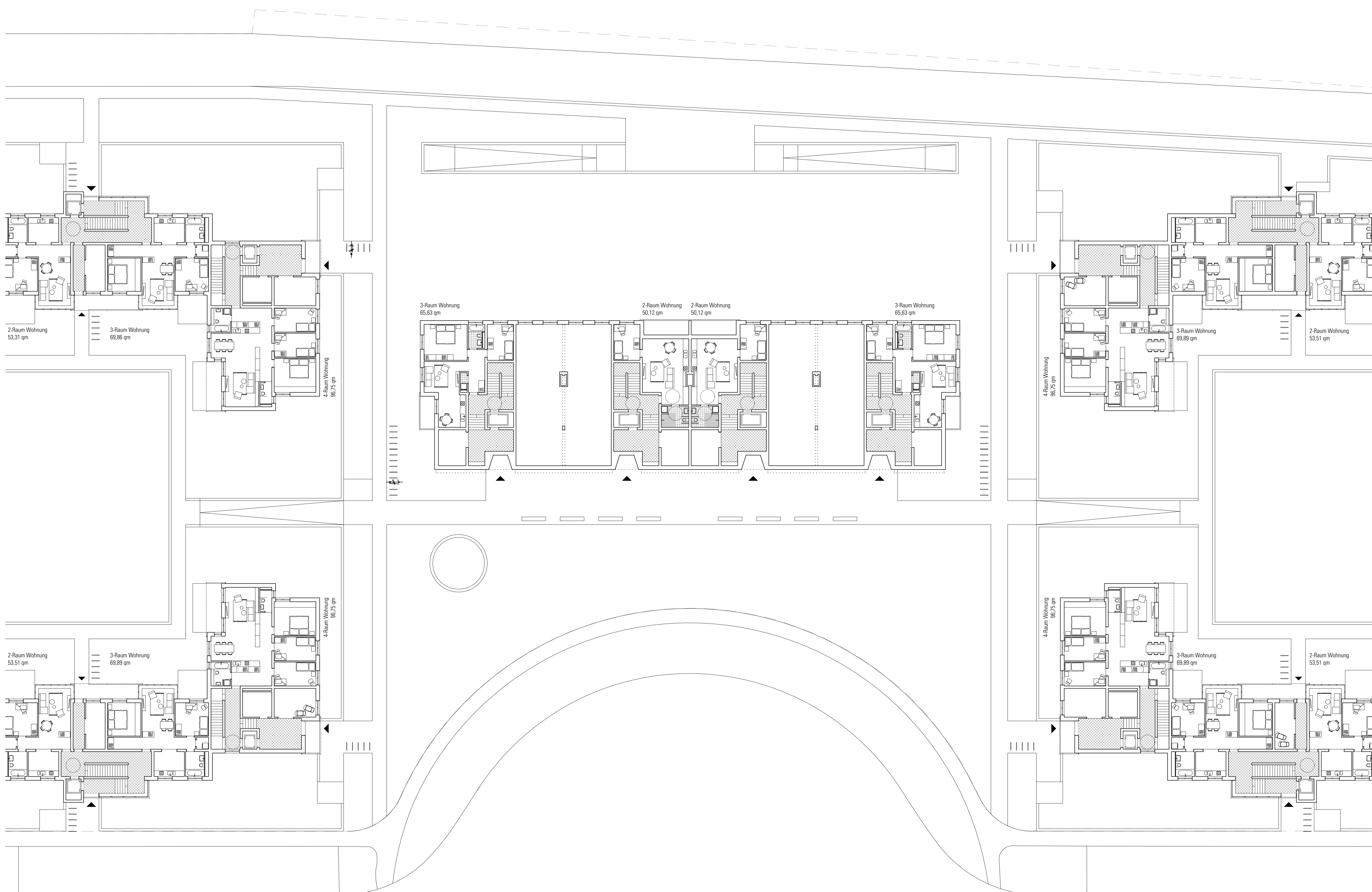
Erdgeschoss M 1:200
