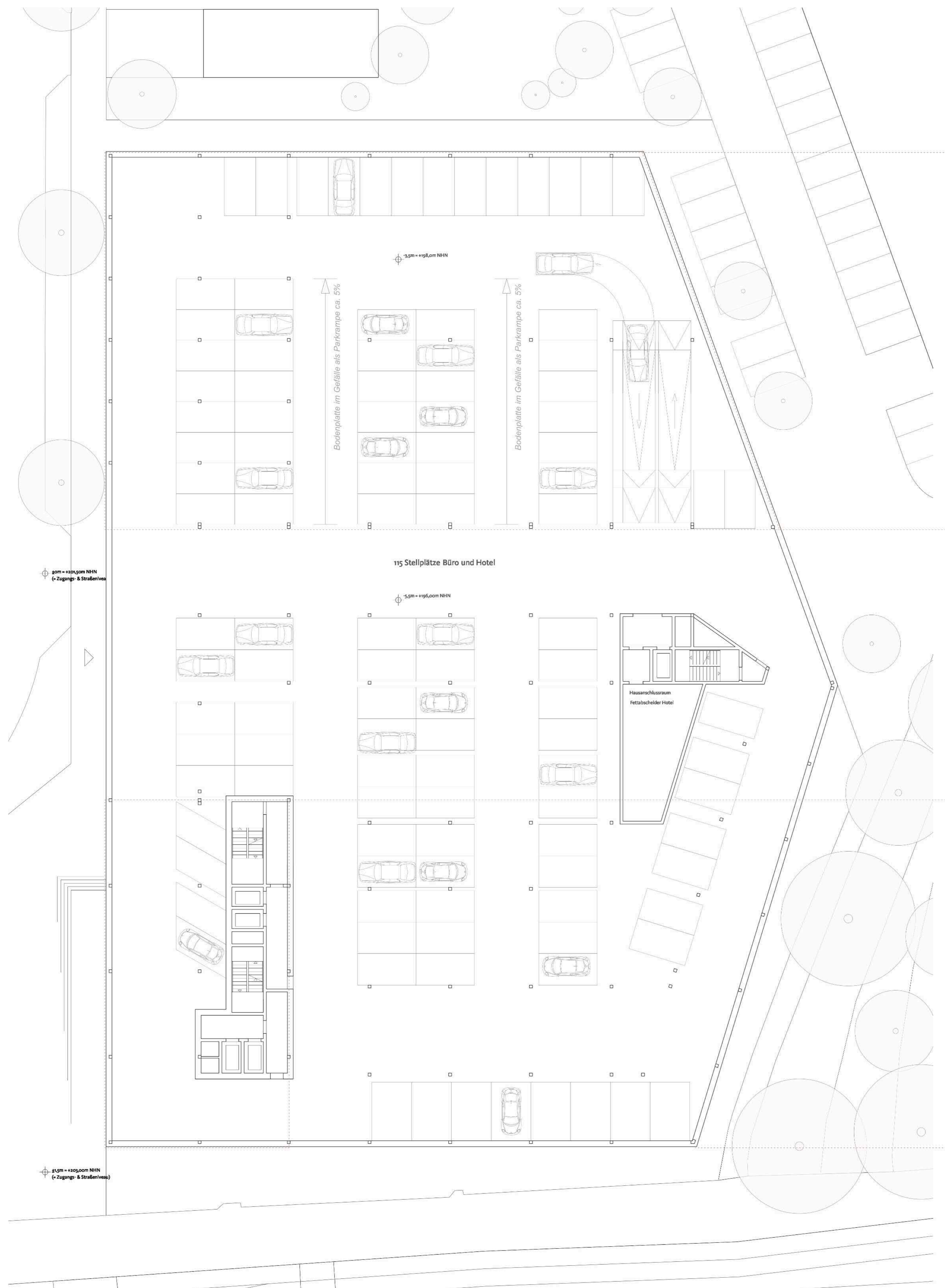
GRUNDRISS UNTERGESCHOSS M 1:200
