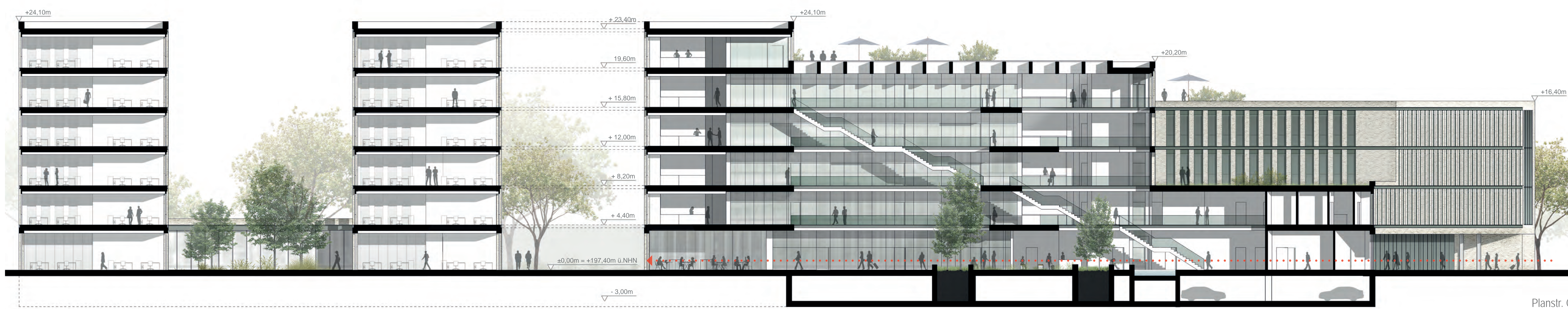
Innenhof Bahngasse Atrium 1f.Längsschnitt A-A 1:200
