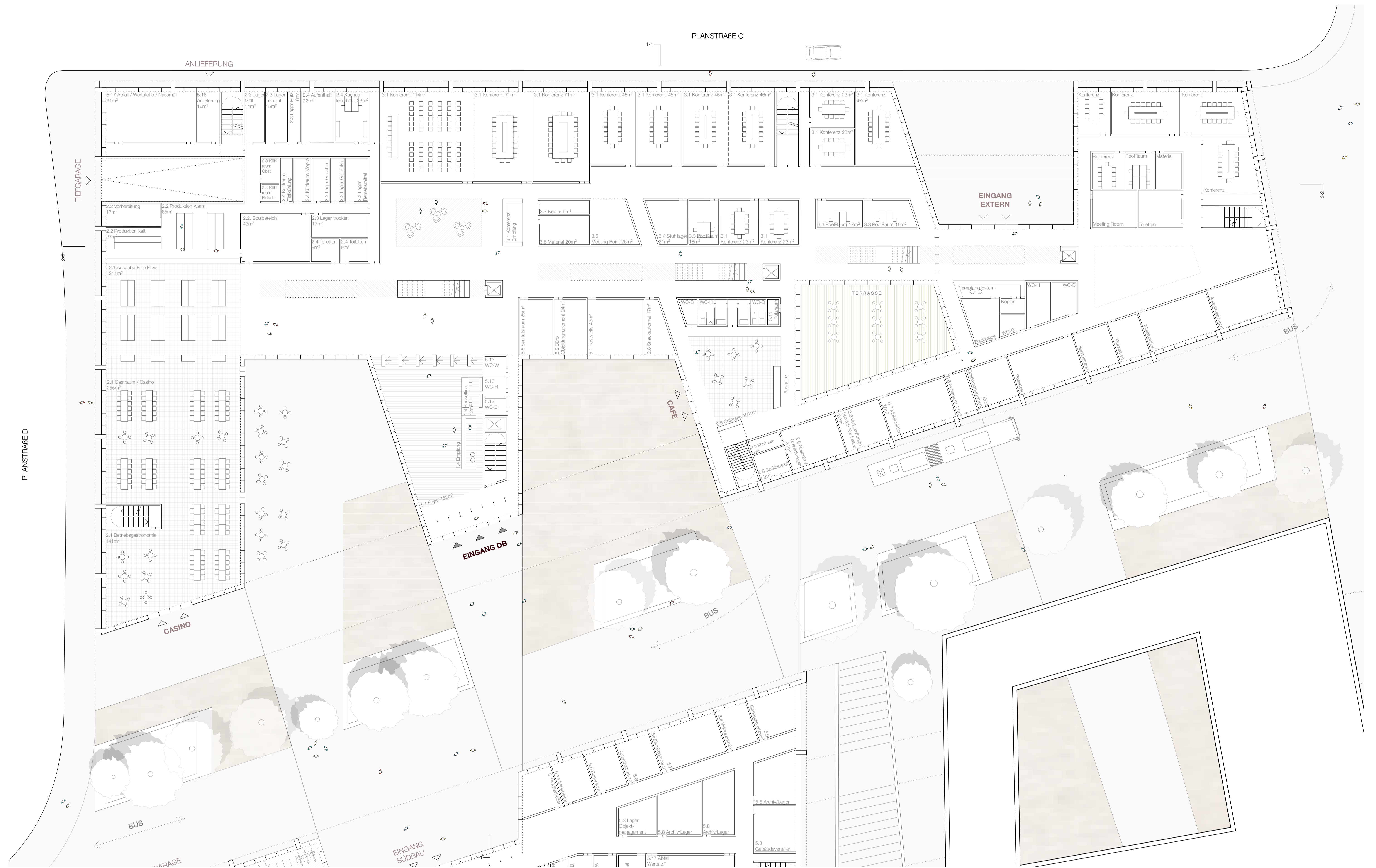
ERDGESCHOSS BAUFELD NORD M1:200
